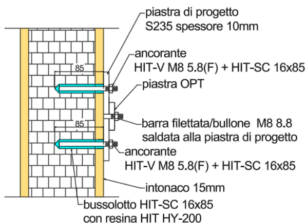
Figura 1 – Sezione dell'ancoraggio al muro
