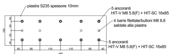
Piastra di progetto a cui viene collegata la piastra OPT
